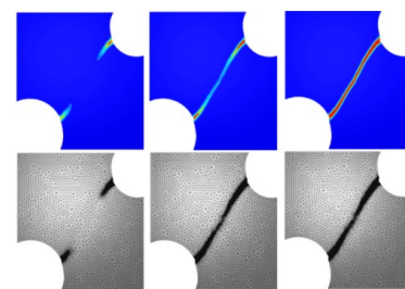
Simulation de l'amorçage et de la propagation d'une fissure
